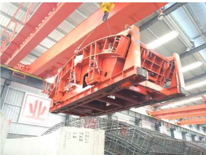
地铁管片
